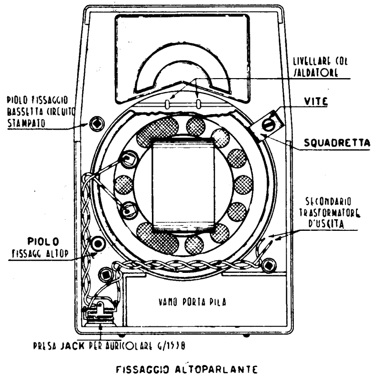
Montaggio del jack e dell'altoparlante nel mobiletto.
